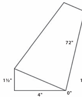
Wedge #12
